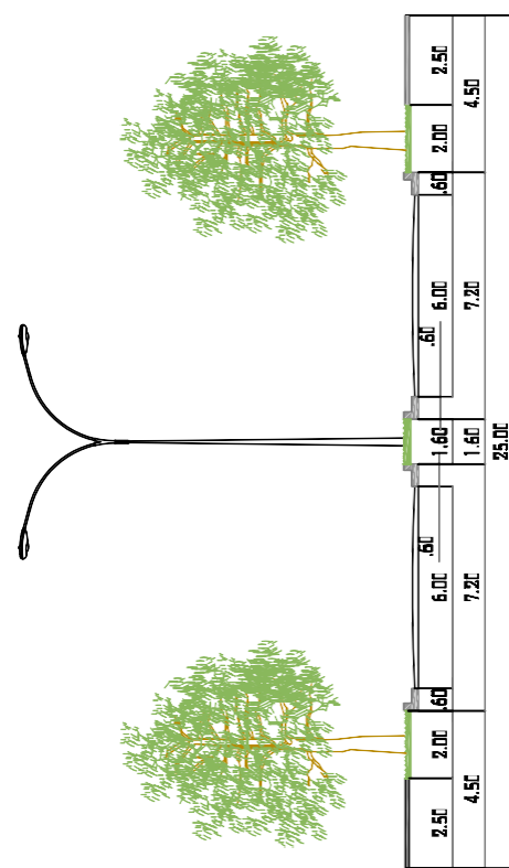
PERFIL 3 VIA ESTRUTURAL
