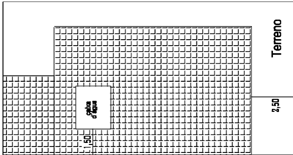
DETALHE 3 - LOCAÇÃO
