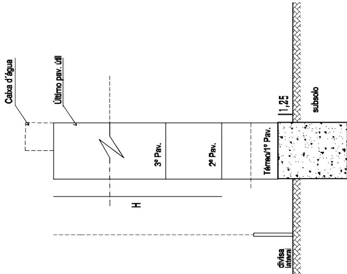
DETALHE 1 - CORTE ESQUEMÁTICO
